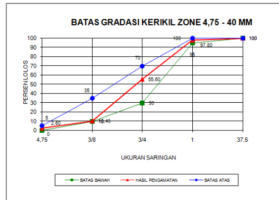
Gambar 2. Hubungan ukuran saringan dengan persen lolos kerikil/batu pecah
