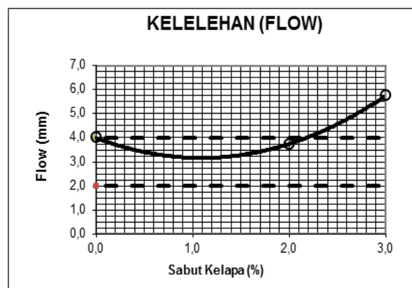
Gambar 5. Grafik Hubungan Sabut Kelapa dan Kelelehan ( Flow )
