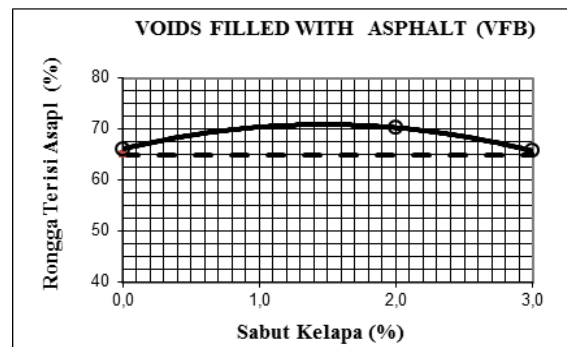
Gambar 10. Grafik Hubungan Sabut Kelapa dan VFB
