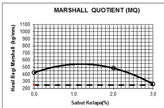
Gambar 6. Grafik Hubungan Sabut Kelapa dan Marshall Quotient
