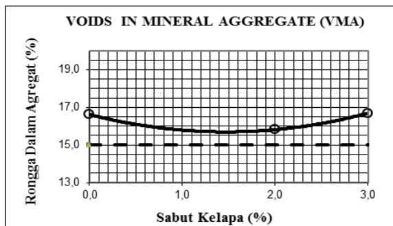
Gambar 9. Grafik Hubungan Sabut Kelapa dan VMA
