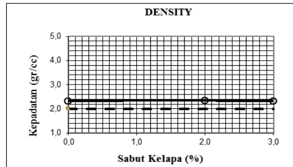
Gambar 7. Grafik Hubungan Sabut Kelapa dan Kepadatan ( Density )
