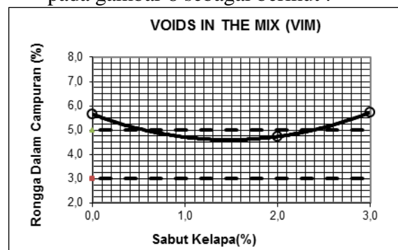
Gambar 8. Grafik Hubungan Sabut Kelapa dan VIM
