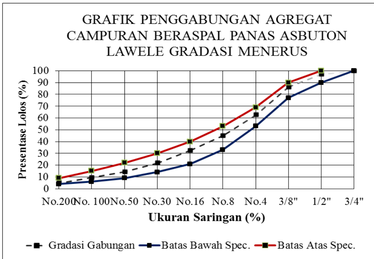
Gambar 3. Grafik Gabungan Agregat Campuran Laston Lapis Aus (AC-WC)
