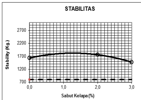
Gambar 4. Grafik Hubungan Sabut Kelapa dan Stabilitas
